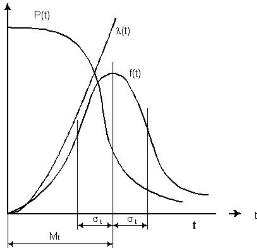
Кривые нормального закона распределения
