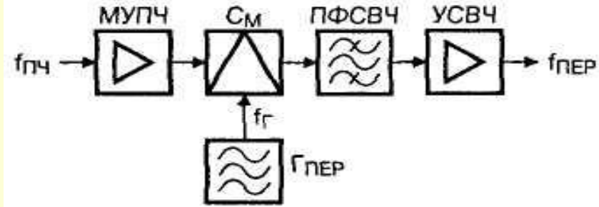
Рис. 2. Функциональная схема передатчика радиоствола.
