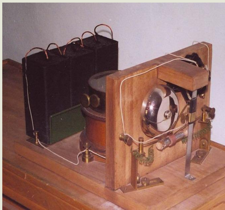
Радиоприемник Попова. 1895г. Копия. Политехнический музей. Москва.
