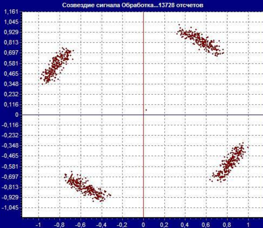
Сигнальное Созвездие - Constellation
