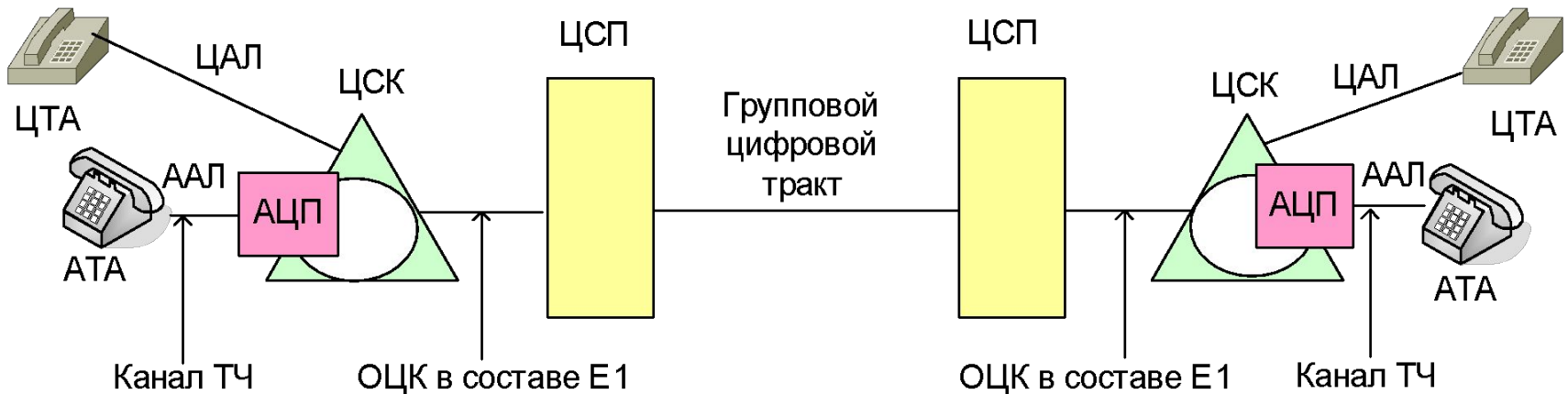
Цифровая телефонная сеть с использованием каналов ОЦК
