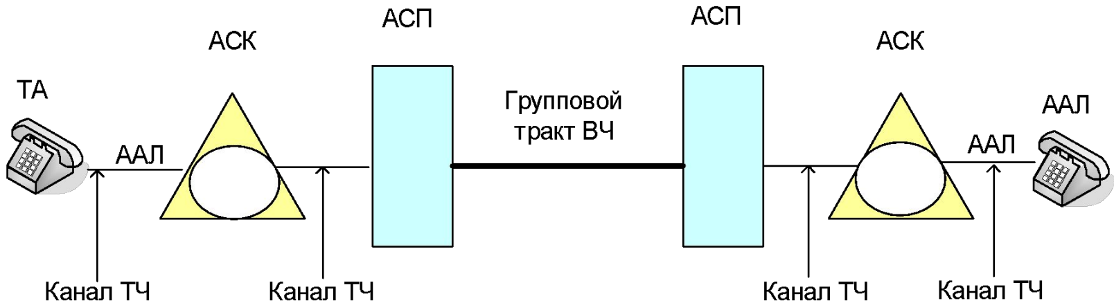
Аналоговая телефонная сеть с использованием каналов КТЧ
