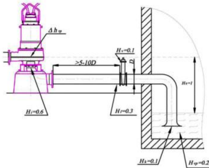
Рис. 2. Расчет геометрической высоты всасывания H_{0\text{г}}
