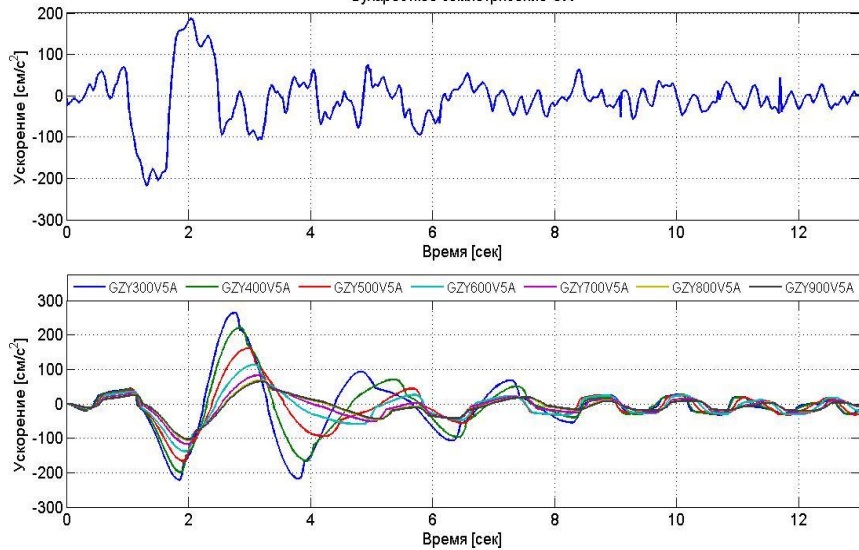
Исходная акселерограмма (вверху) и модифицированные сигналы (внизу) для разных типоразмеров РМО.
