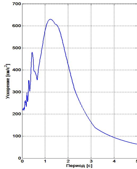
Спектр реакции исходной акселерограммы (слева) и спектры реакции модифицированных сигналов (справа) для разных типоразмеров РМО. Землетрясение в г.Бухарест ОХ. Двухмассовая система
