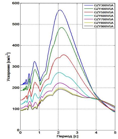
Спектр реакции исходной акселерограммы (слева) и спектры реакции модифицированных сигналов (справа) для разных типоразмеров РМО. Землетрясение в г.Бухарест ОХ. Двухмассовая система
