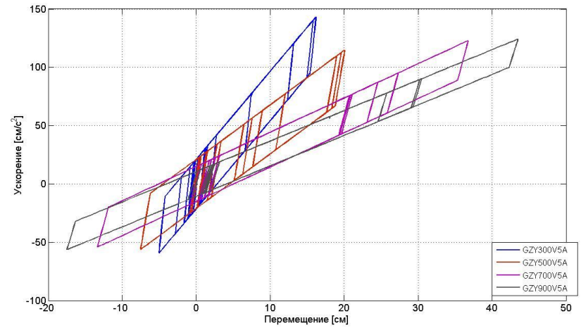
Диаграммы зависимости «Ускорение- Перемещение» в верхней части сейсмоопоры для разных типоразмеров РМО. Землетрясение в г.Газли ОХ.
