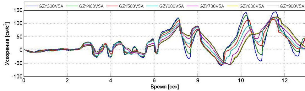
Исходная акселерограмма (вверху) и модифицированные сигналы (внизу) для разных типоразмеров РМО. Землетрясение в г.Газли ОХ.
