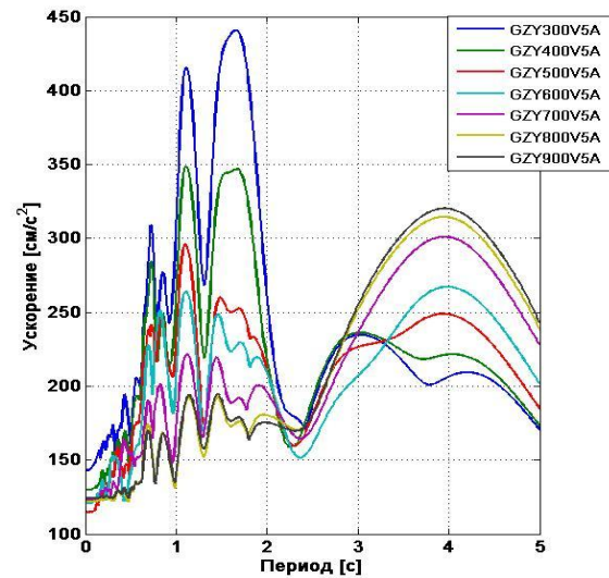
Спектр реакции исходной акселерограммы (слева) и спектры реакции модифицированных сигналов (справа). Землетрясение в г.Газли ОХ.
