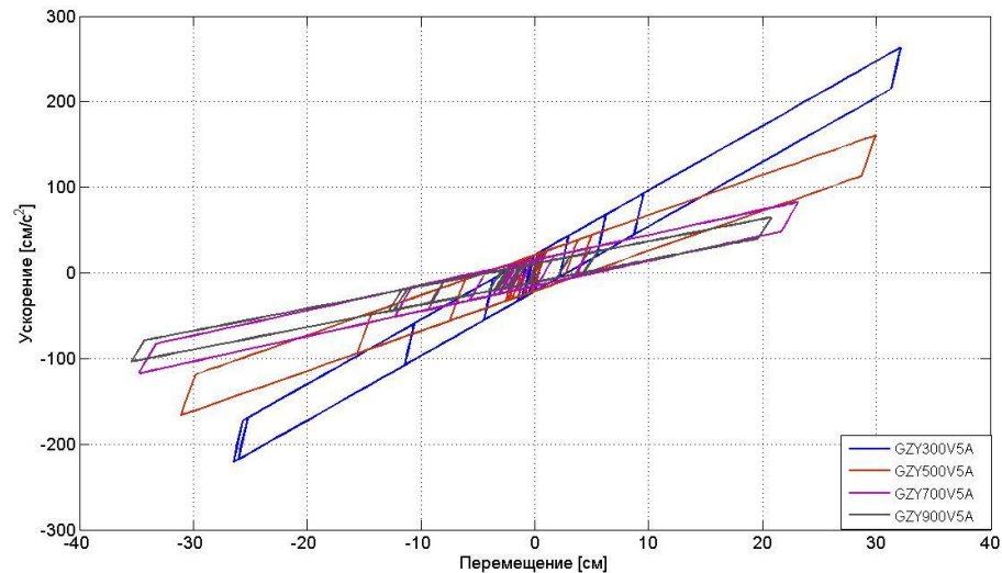
Диаграммы зависимости «Ускорение- Перемещение» Одномассовая система. Землетрясение Бухарест ОХ.
