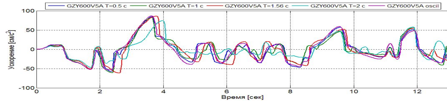
Исходная акселерограмма (вверху) и модифицированные сигналы (внизу) для разных характеристик верхней части системы. Землетрясение в г.Эль-Центро ОУ.
