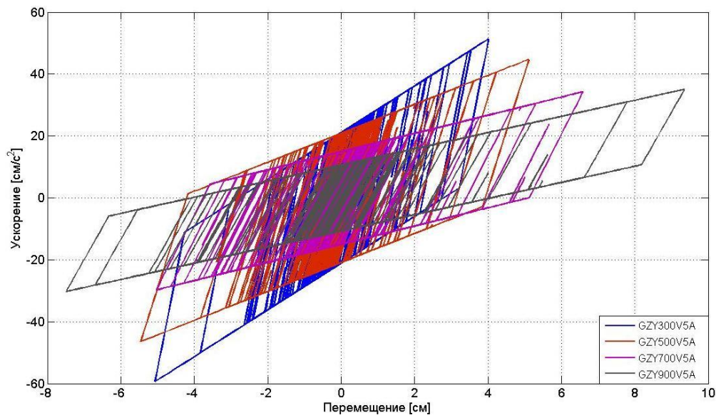
Диаграммы зависимости «Ускорение- Перемещение» для разных типоразмеров РМО. Одномассовая система. Землетрясение в Японии 11.03.2011 ОХ.
