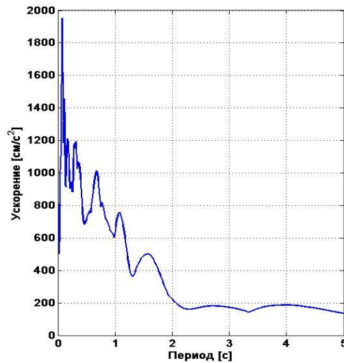
Спектр реакции исходной акселерограммы (слева) и спектры реакции модифицированных сигналов (справа). Землетрясение в г.Газли ОХ.
