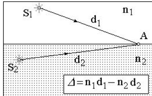
Рис. 2.3 Оптическая разность хода.
