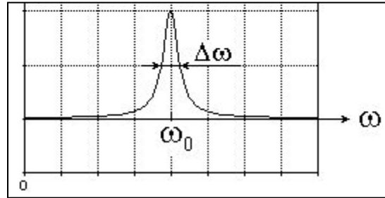
Рис. 2.2 Ширина спектра излучения
