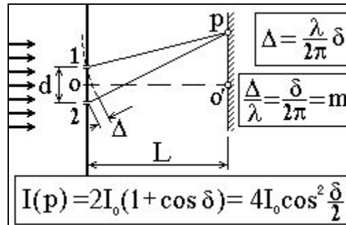
Рис. 2.4 Интерференция двух монохроматических волн: источники – две щели в непрозрачной экране, освещаемом плоской волной
