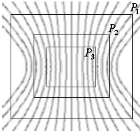
Рис. 2.4 Двумерная интерференционная картина
