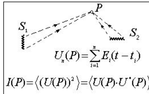
Рис. 2.1 Принцип суперпозиции
