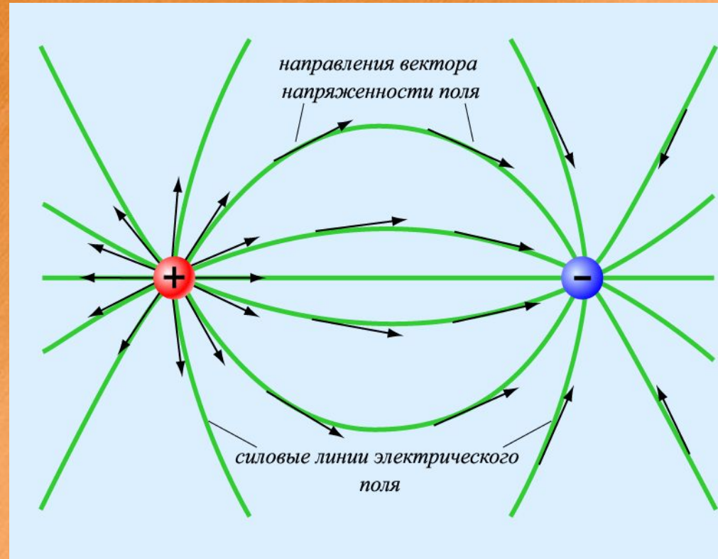
Рис 1. Электростатическое поле для 2-х заряженных тел
