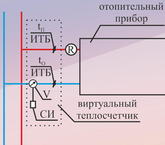
Двухтрубная система отопления
