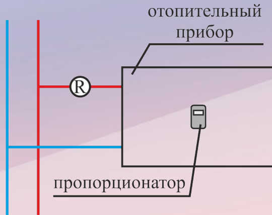
Двухтрубная система отопления
