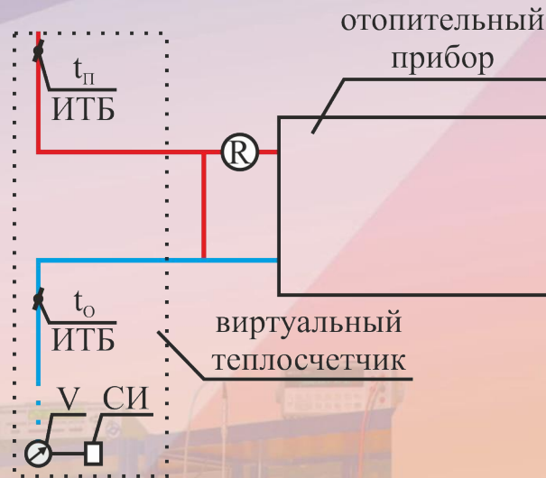
Однотрубная система отопления
