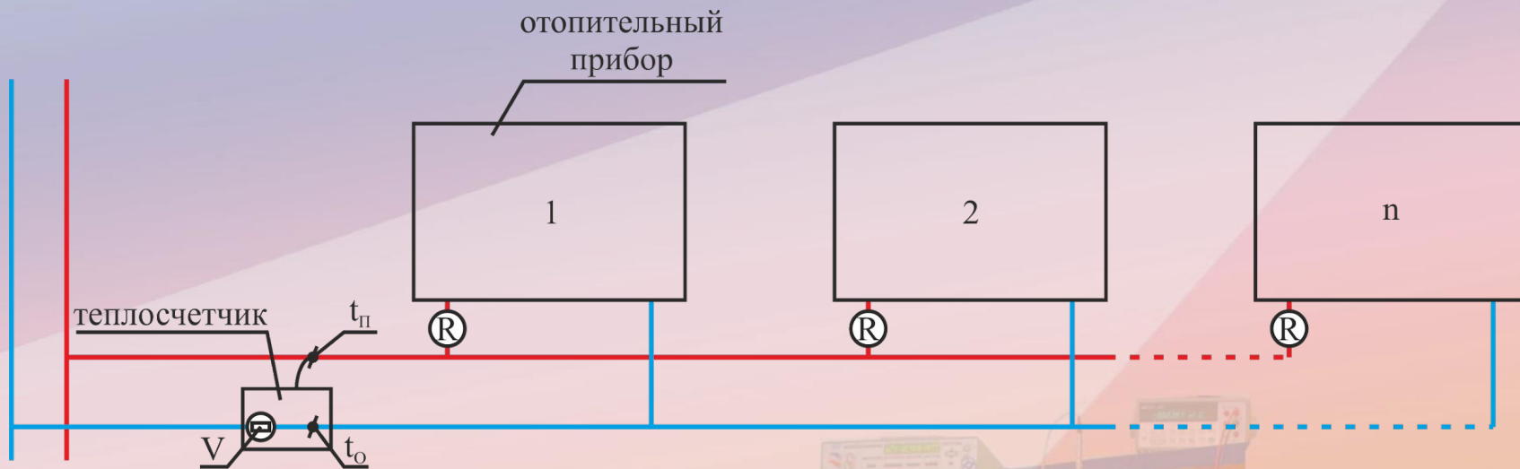
Двухтрубная горизонтальная система отопления
