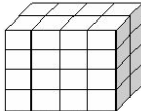
ТРЕХМЕРНЫЙ МАССИВ
