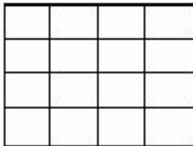
ДВУМЕРНЫЙ МАССИВ
