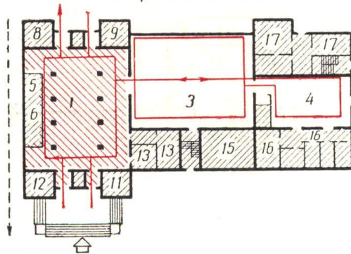
Первый этаж
