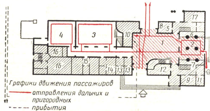
Первый этаж
