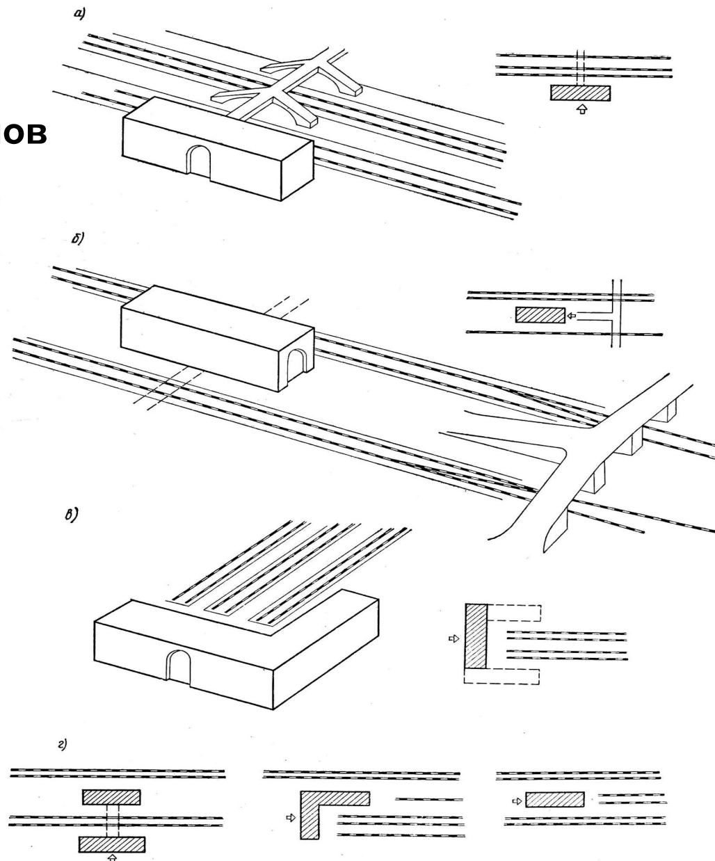
Типы железнодорожных вокзалов в зависимости от расположения здания по отношению к при- станционным путям
