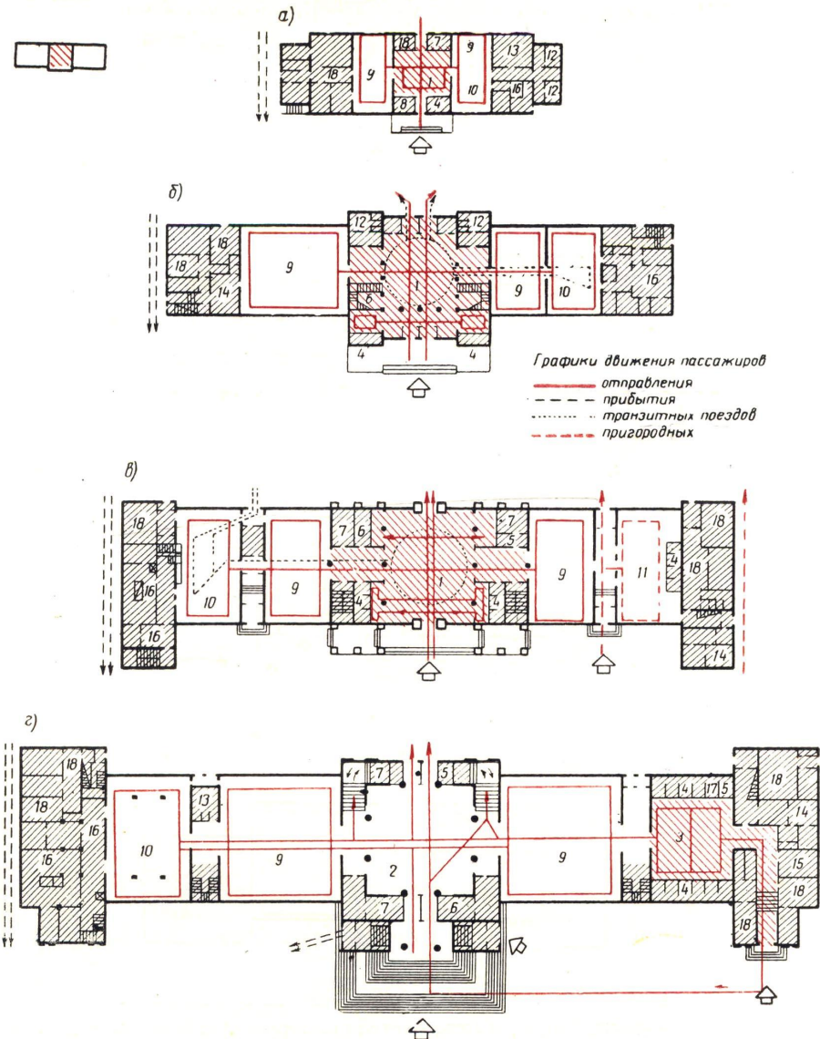
а — типовой проект вокзала на 100 человек; б — вокзал в Ржеве; в — вокзал в Запорожье; г — вокзал в Волгограде; 1 — вестибюль — операционный зал; 2 — распределительный зал; 3 — кассовый зал; 4 — кассы; 5 — справочное бюро; 6 — почта, телеграф; 7 — кабинет начальника вокзала и дежурного; 8 — камера хранения; 9 — зал ожидания; 10 — ресторан, буфет; 11 — пригородный зал; 12 — санитарный узел; 13 — комната матери и ребенка; 14 — медпункт; 15 — милиция; 16 — кухня ресторана; 17 — касса аэрофлота; 18 — прочие помещения
