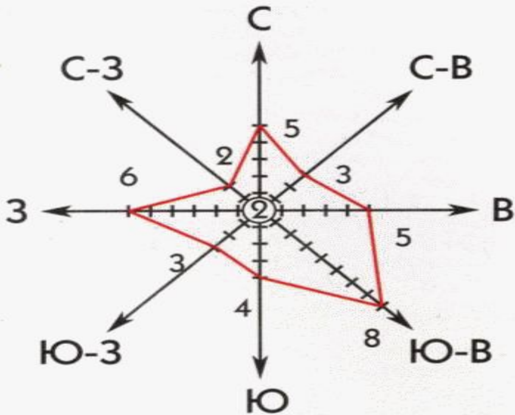
Роза ветров
