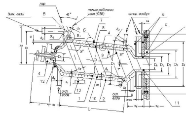
Конструкция термоциклонного предтопка (ТЦП) горизонтального типа мощностью 25 и 50 МВт
