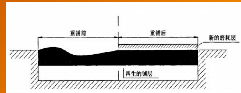
重铺再生
