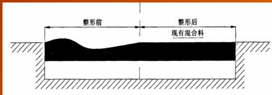
整形再生
