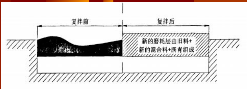
复拌再生
