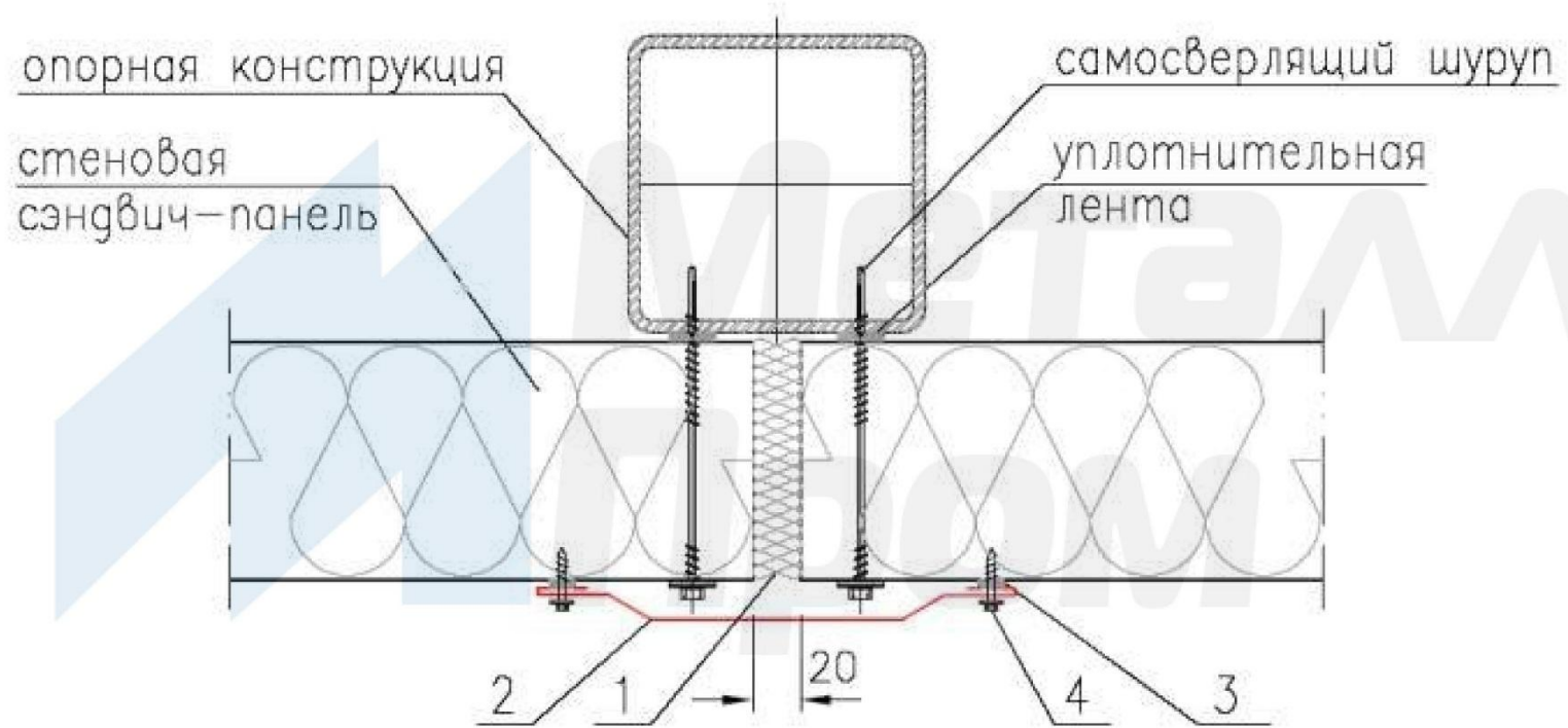
Рис.10. Поперечный стык стеновых панелей
