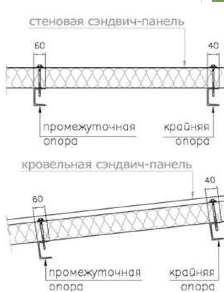
Рис.5 Опорные конструкции
