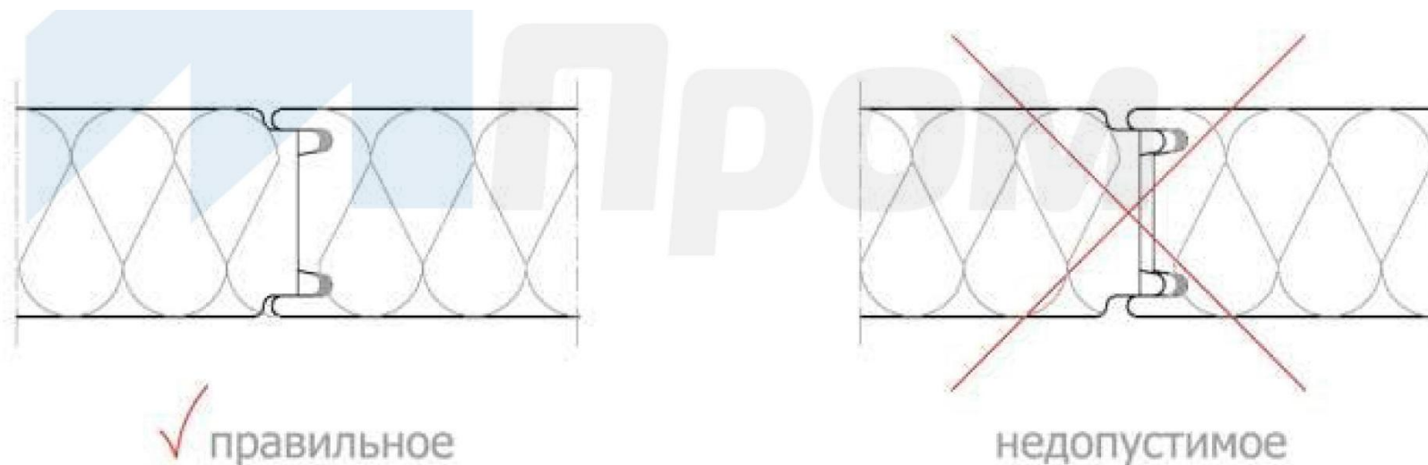
Рис.8. Соединение стеновых панелей между собой
