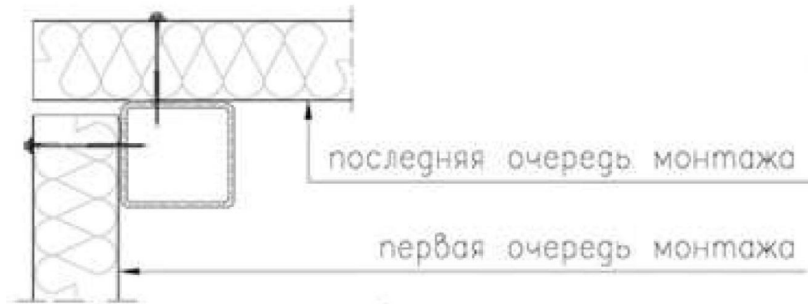
Рис.6. Схема порядка монтажа угловых панелей
