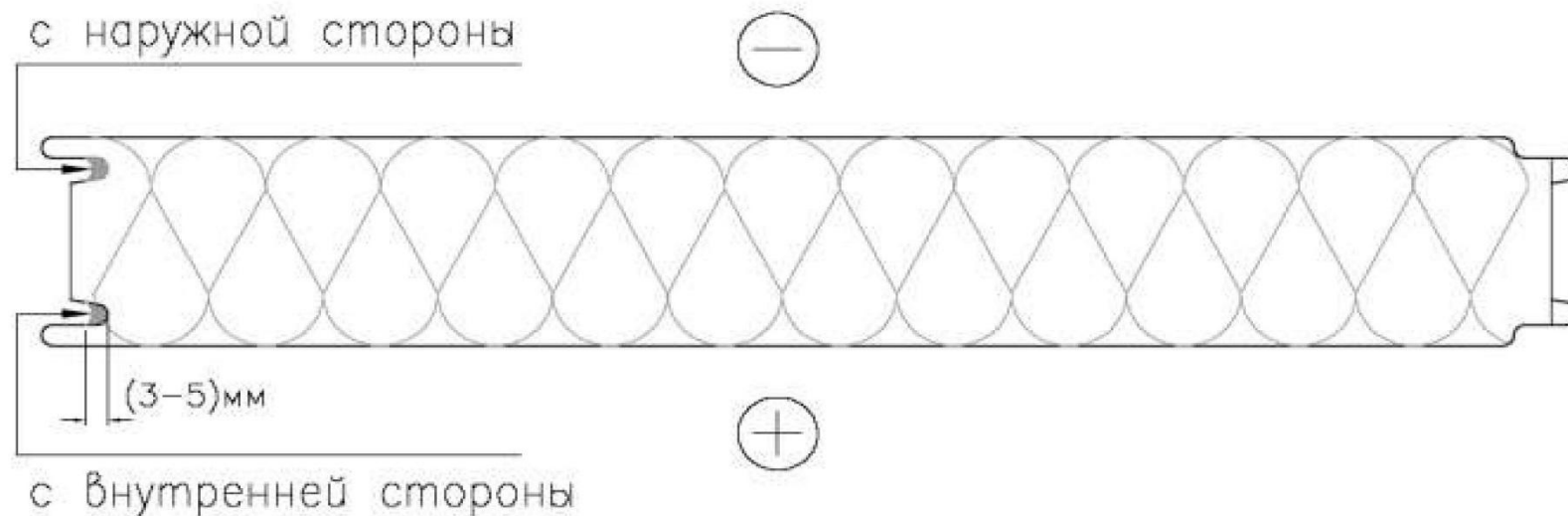
Рис.9. Закладка герметика в замок стеновой панели
