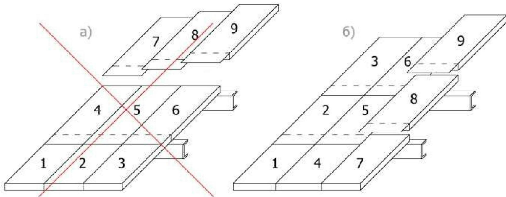
Рис.11. Схема раскладки кровельных сэндвич панелей
