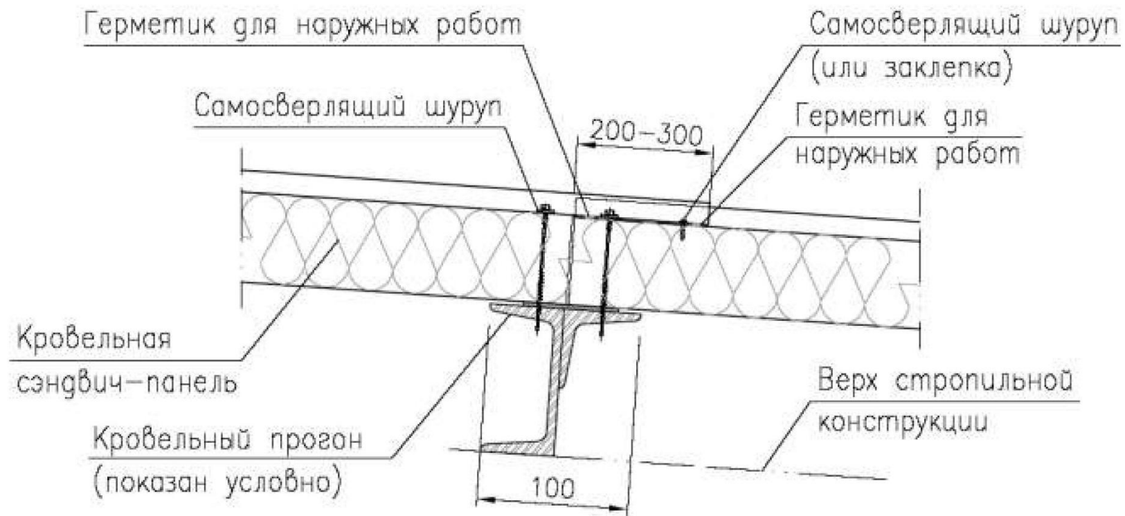
Рис. 13. Нахлест кровельных панелей. Окончание монтажа
