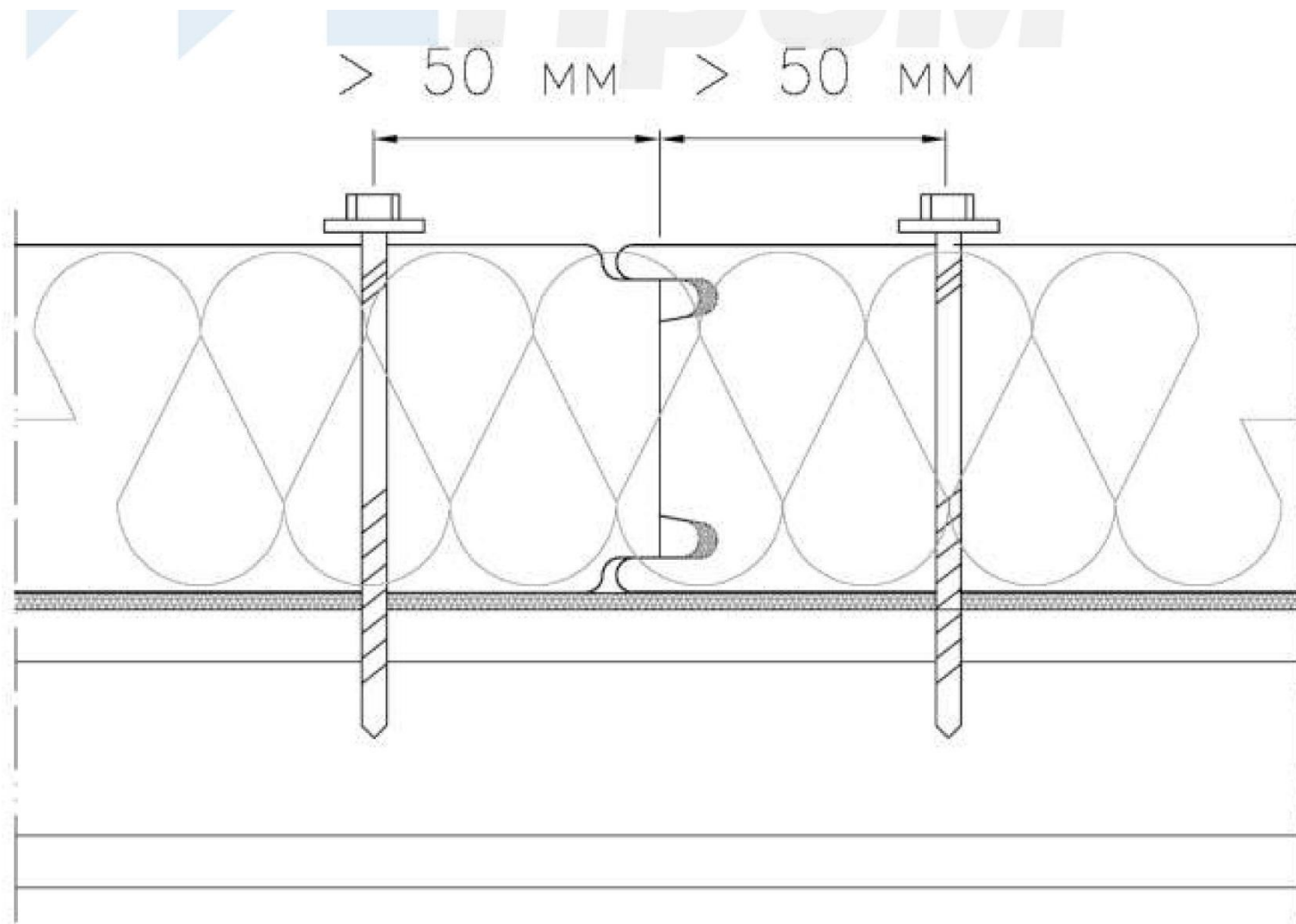
Рис.3. Крепление панелей к подконструкции
