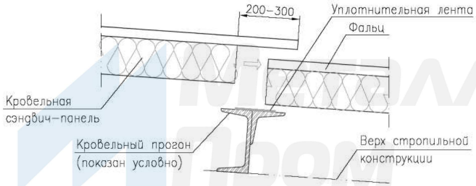
Рис. 12. Нахлест кровельных панелей. Начало монтажа
