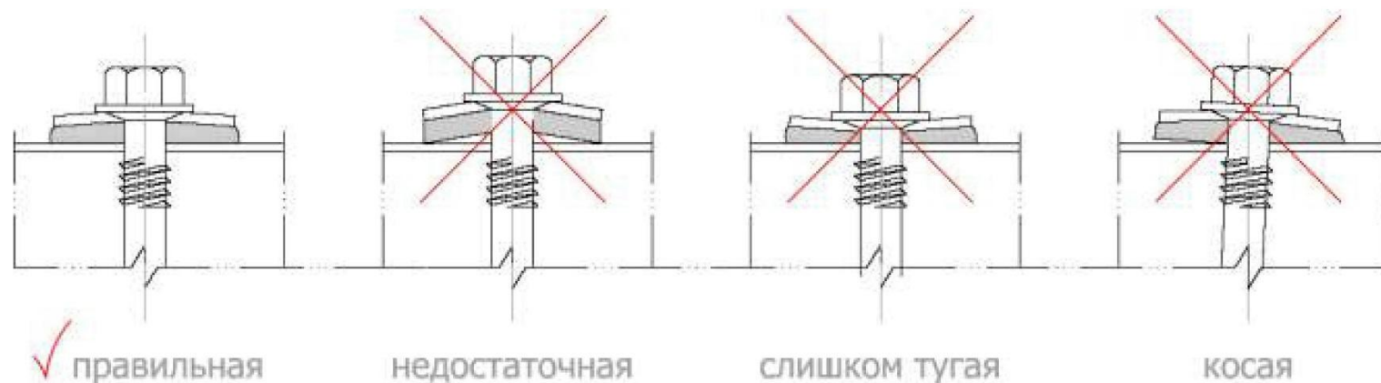
Рис.4 Посадка шурупов
