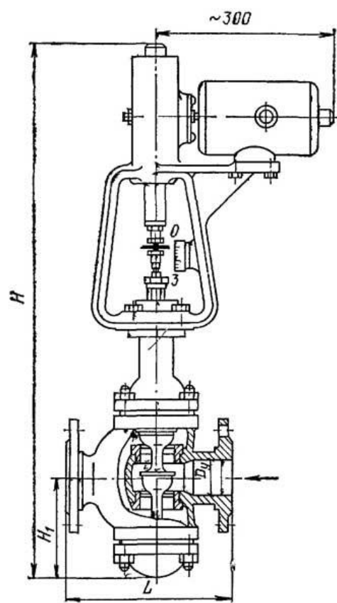
Рис. 48. Клапан регулирующий с электрическим исполнительным механизмом 25ч931нжНО
