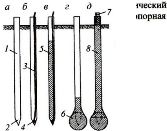
Рис. 2.16. Технологическая схема А. А. Луги для изготовления свай с камуфлетной пятой:
