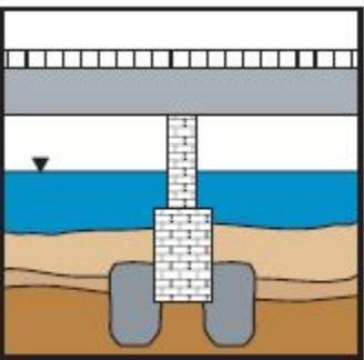
Закрепление грунтов основания по периметру фундаментов
