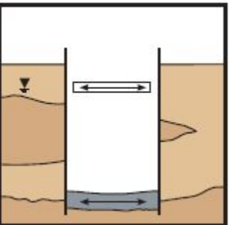
Устройство распорных плит ниже дна котлована
