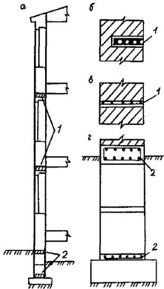
Устройство поясов армирования: а – размещение поясов в стене по вертикали; б – железобетонный пояс; в – армированный пояс в утолщенном шве кладки; з – размещение пояса по обрезу фундамента
