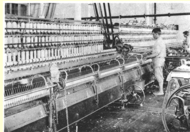
Мельно-пряльное отделение.
