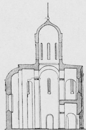
Продольный разрез
