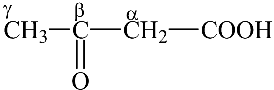
3-оксобутановая (ацетоуксусная) кислота
