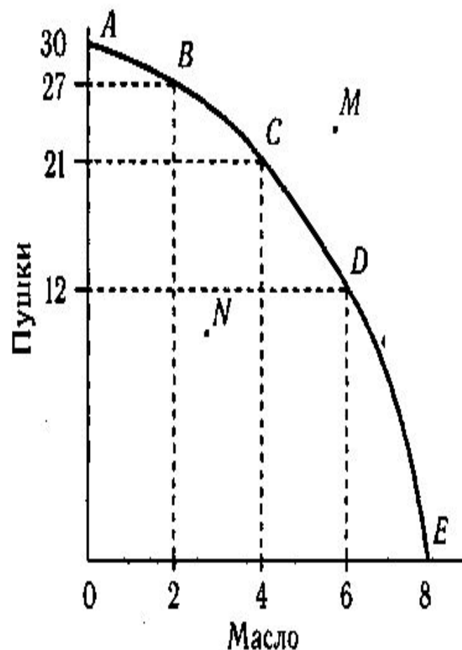
Рис. 1.2. Кривая производственных возможностей
