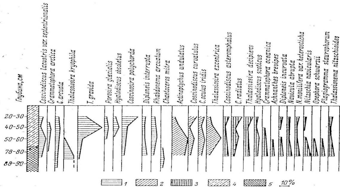
Рис. 2. Распределение доминантных и характерных видов в последнедевических донных осадках северной части Белого моря (Забелина, 1969).
