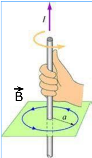
Правило буравчика для магнитной индукции (индукции магнитного поля)
