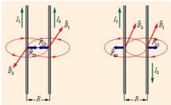
Магнитное взаимодействие параллельных и антипараллельных токов
