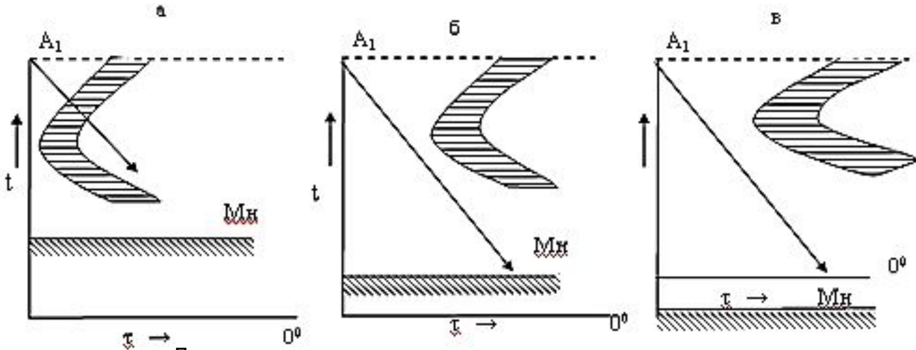
Диаграмма изотермического распада аустенита для сталей перлитного (а), мартенситного (б) и аустенитного (в) классов.
