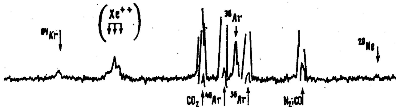
Рис. 2. Фрагмент масс-спектра в области 20–105 а.е.м., полученного в режиме анализа инертных газов с повышенной чувствительностью («Венера-11»)
