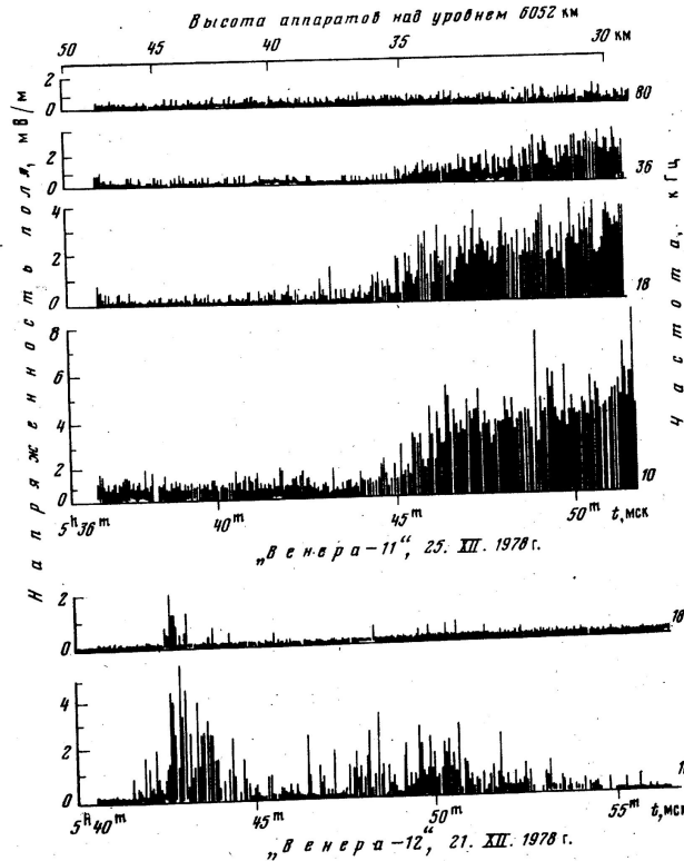
Рис. 2. Радиопульсы импульсного характера, зарегистрированные «Венерой-11» (четыре верхние дорожки) и «Венерой-12» (две нижние дорожки) в функции времени измерений. При спуске в близко расположенных экваториальных районах грозовая активность в случае «Венеры-11» была намного выше Напряженность поля указана для полной полосы частот каждого из каналов. Вверху — высоты аппаратов над точкой посадки
