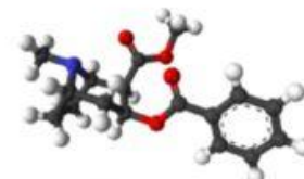
Кокаин
