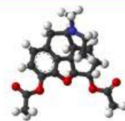
Героин
