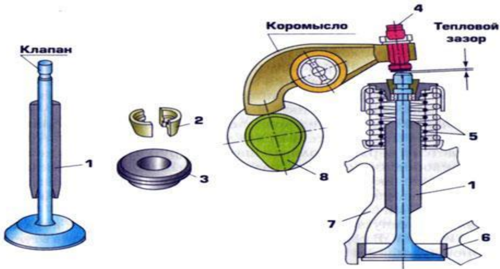
1 — втулка; 2 — сухарь; 3 — шайба; 4 — регулировочный винт; 5 — пружины; 6 — седло клапана; 7 — головка цилиндров; 8 — кулачок распределительного вала;
