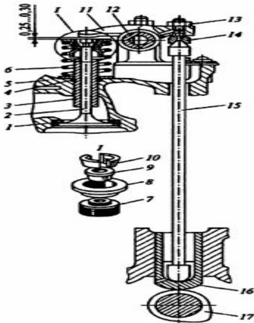
Рис. 3.1. Схема газораспределительного механизма с верхним расположением клапанов:
