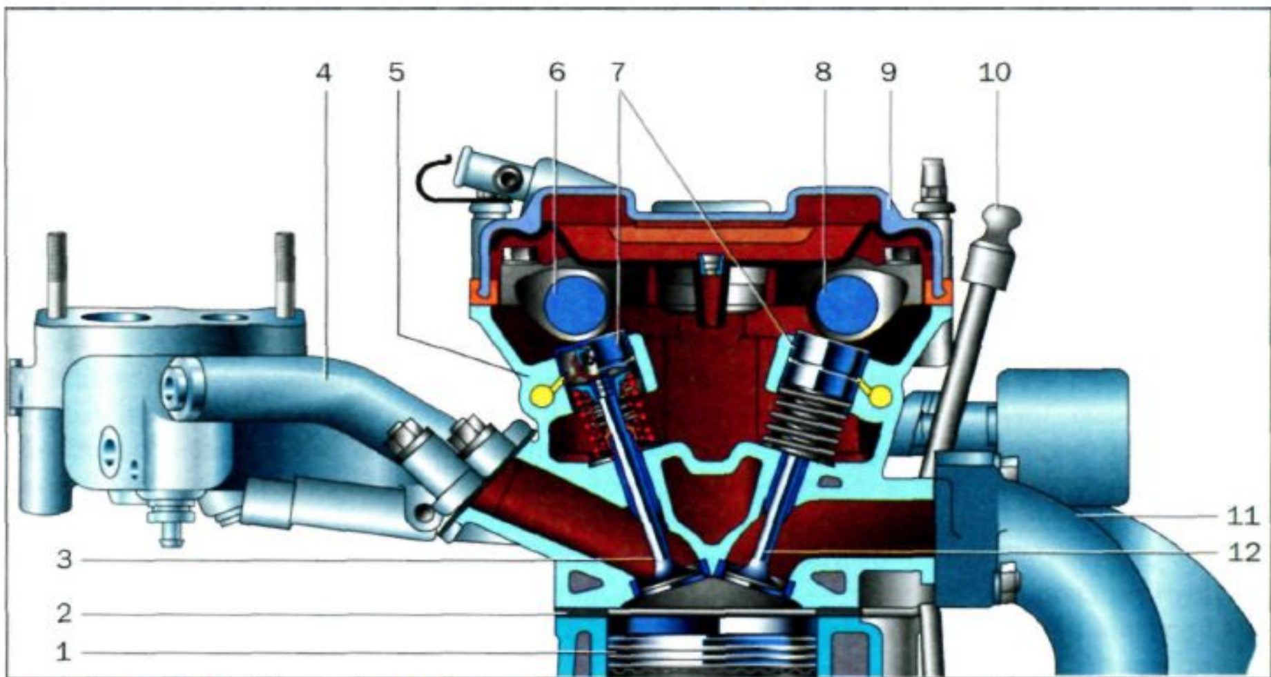
Рис. 2.32 б. ГРМ двигателя 3МЗ-4063: 1 — поршень; 2 — прокладка головки блока цилиндров; 3 — впускной клапан; 4 — впускной трубопровод; 5 — головка блока цилиндров; 6 — распределительный вал впускных клапанов; 7 — гидротолкатели; 8 — распределительный вал выпускных клапанов; 9 — крышка головки блока цилиндров; 10 — масломерный щуп; 11 — выпускной коллектор; 12 — выпускной клапан
