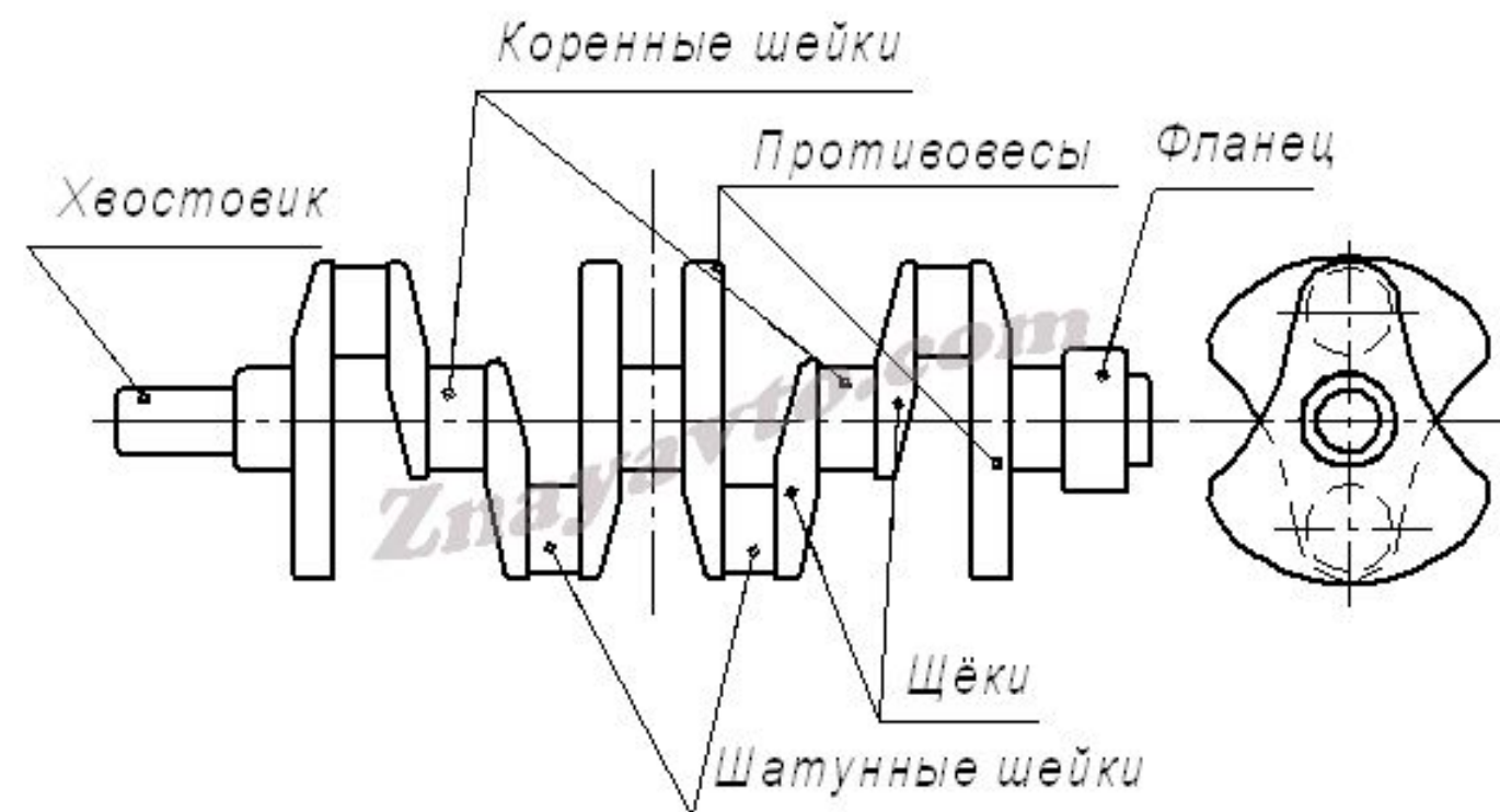
Коленчатый вал рядного четырёхцилиндрового двигателя
