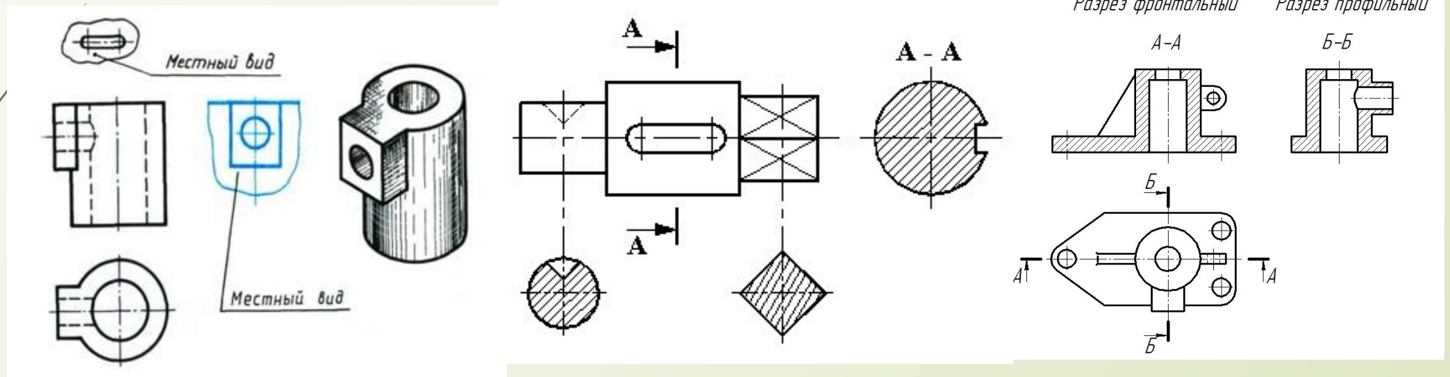
Разрезы
