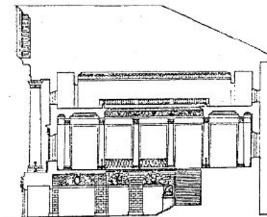
РАЗРЕЗ ВЕСТИБУЛЯ
