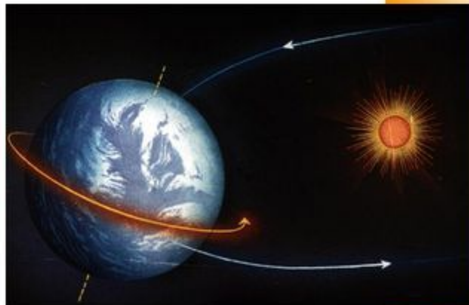
ОРБИТАЛЬНОЕ ВРАЩЕНИЕ
