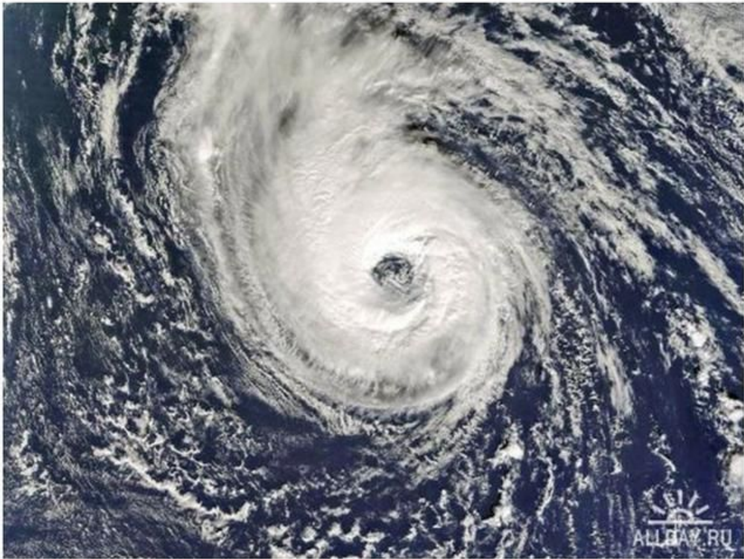
Тайфун Эпсилон
