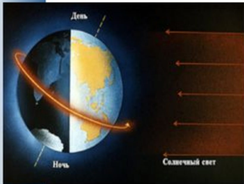
ОСЕВОЕ ВРАЩЕНИЕ
