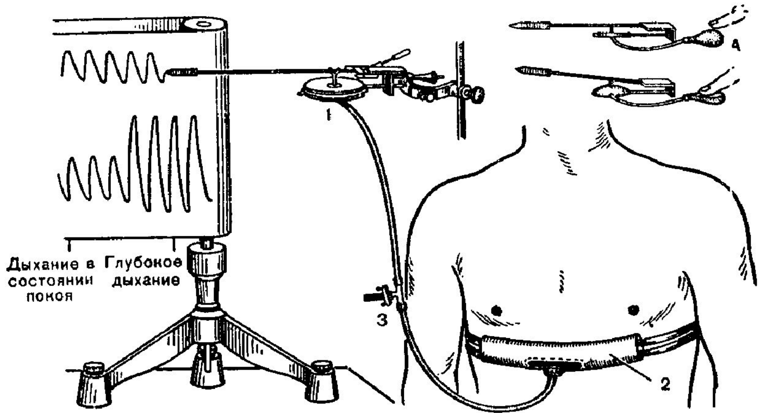
пневмограф Маррея
