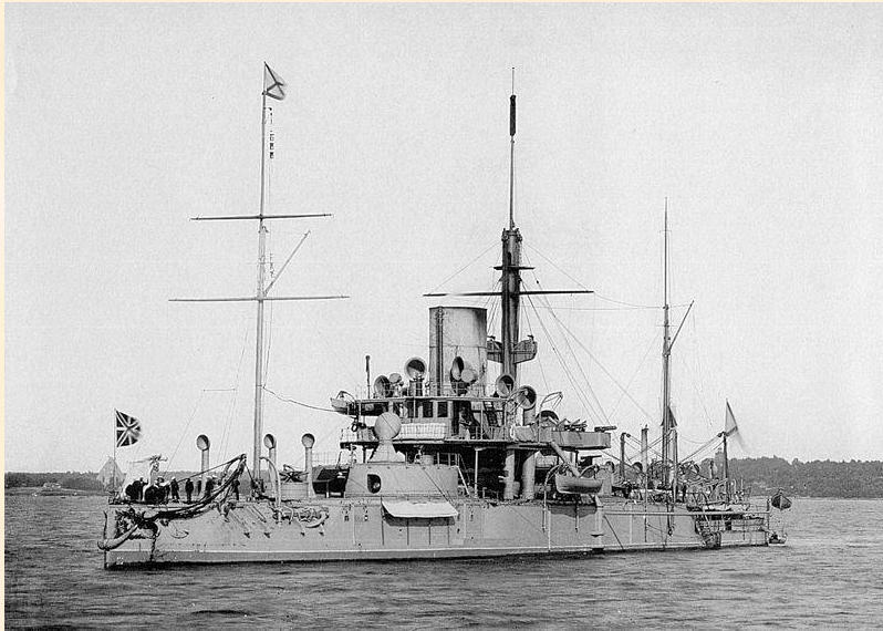
Первый русский броненосец «Петр Великий» (1869 г.)
