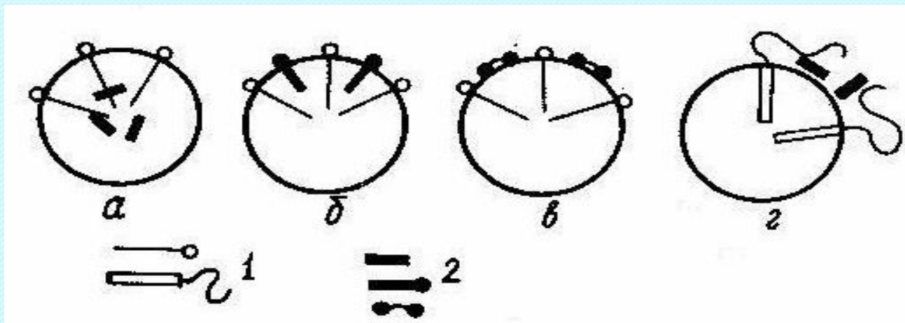
Рис. 2. Солюбилизация в мицеллах ПАВ: неполярных углеводов (а), длинноцепочечных спиртов и аминов (б), полярных веществ (в), ароматических соединений в мицеллах неионного ПАВ (г); 1 — ПАВ, 2 — солюбилизиаты.
