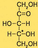
D -ксилулоза
