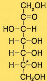
D -седогеπτулоза
