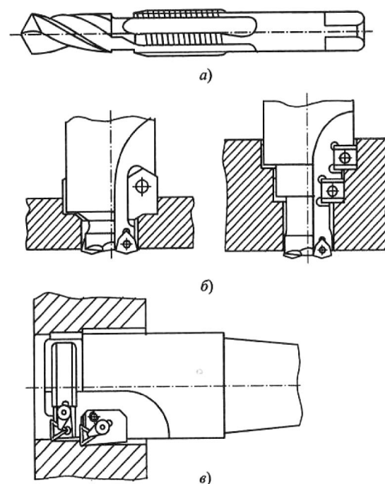
Рисунок 1 - Комбинированные инструменты: а — сверло- метчик; б — сверло-зенкер; в — расточная оправка, оснащенная твердосплавными СМП
