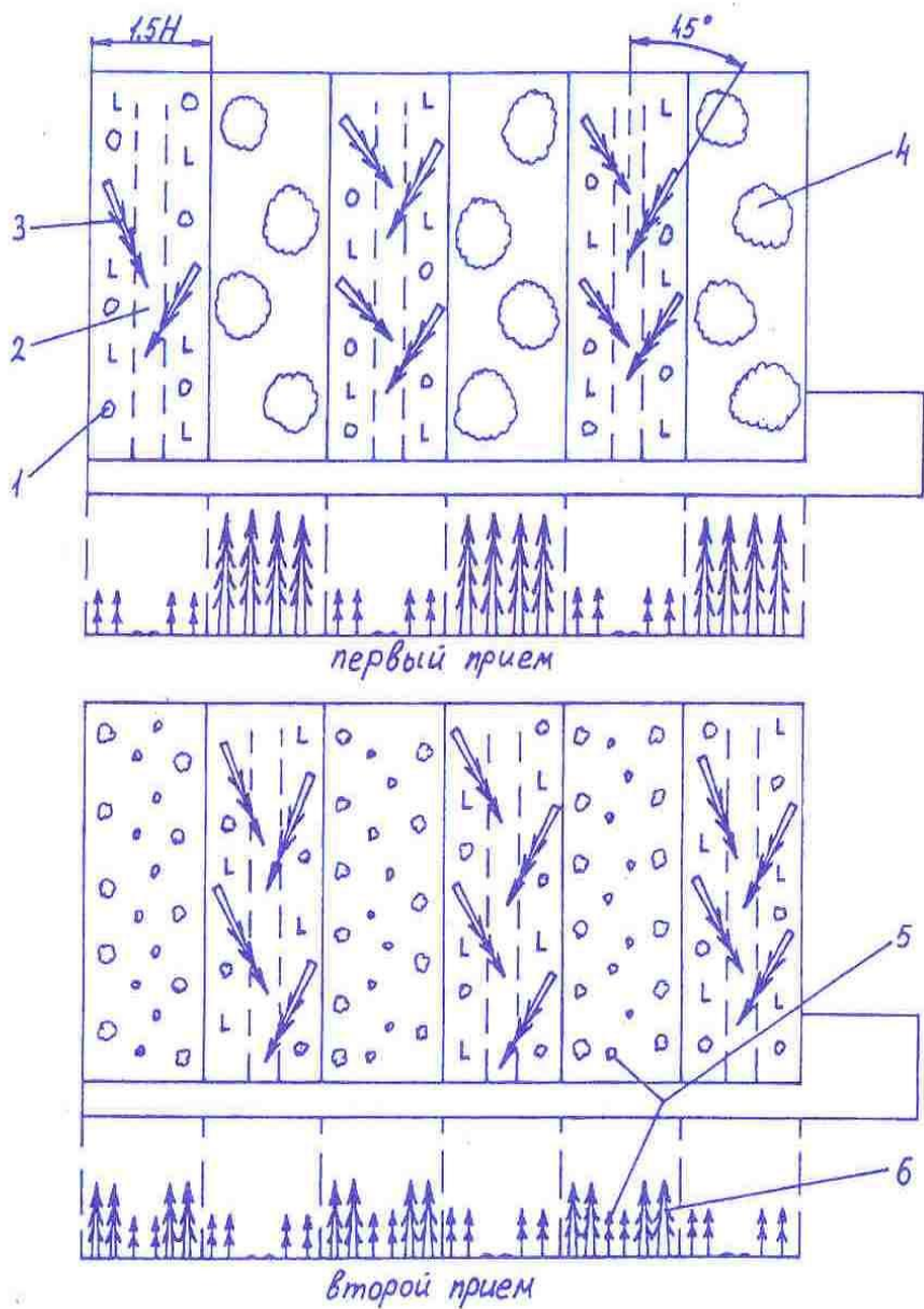
Рис. 16. Схема проведения двухприемной чересполосно-постепенной рубки:
