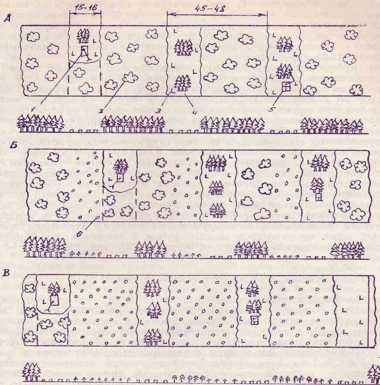
Рис. 14. Схема полосно-постепенных рубок валочно-пакетирующей машиной ЛП-19 и трактором для бесчokerной трелевки А — первый прием рубок, Б — второй прием, В — третий прием 1 — валочно-пакетирующая машина, 2 — растущее дерево, 3 — пень, 4 — пачка деревьев, 5 — трелевочный трактор, 6 — подрост
