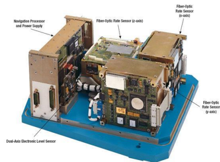
Источники информации о перемещениях судна (акселерометры, гироскопы)
