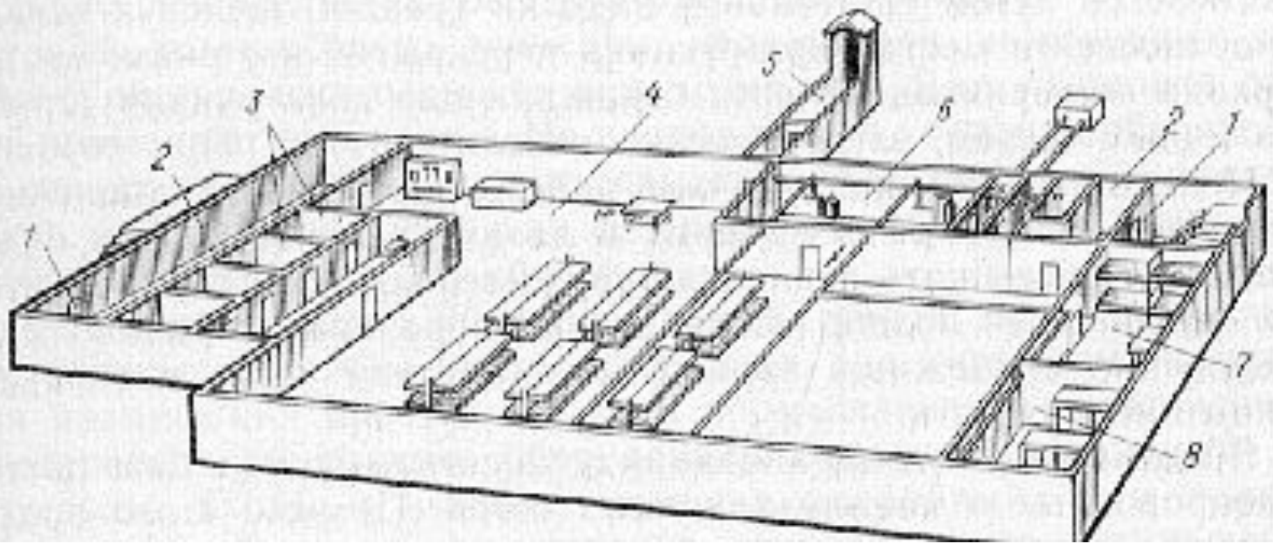
Рис. 89 План убежища
