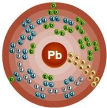
Атом свинца
