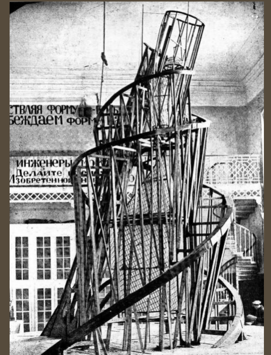
Татлин проект Башни III Интернационала.
