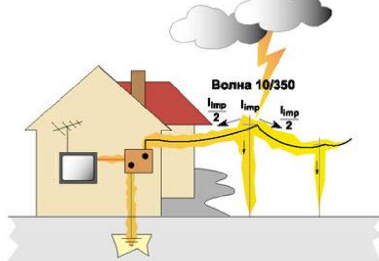
Близкий удар молнии в линию электропередачи
