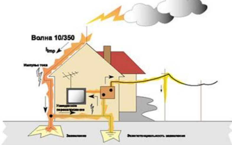
Прямой удар молнии в молниеотвод
