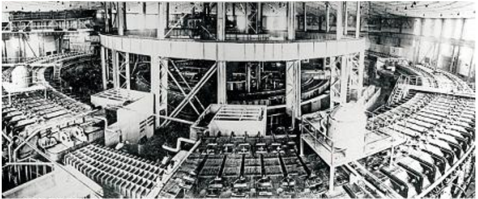
Ярмо магнита синхрофазотрона. Вес электромагнита - 36 тысяч тонн
