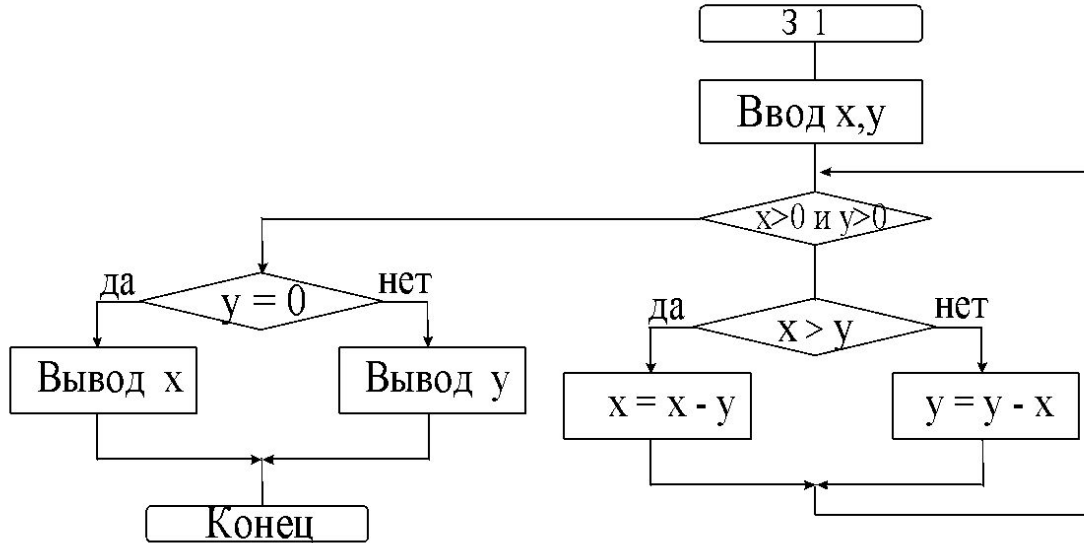
Рис. 8.1. Схема программы 3_1
