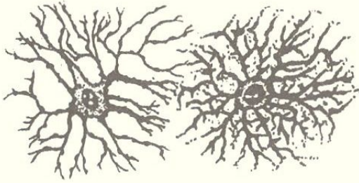
Астроцитарная глия
