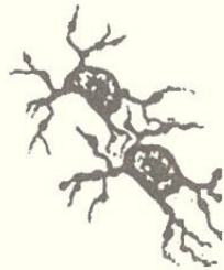
Олигодендроглия
