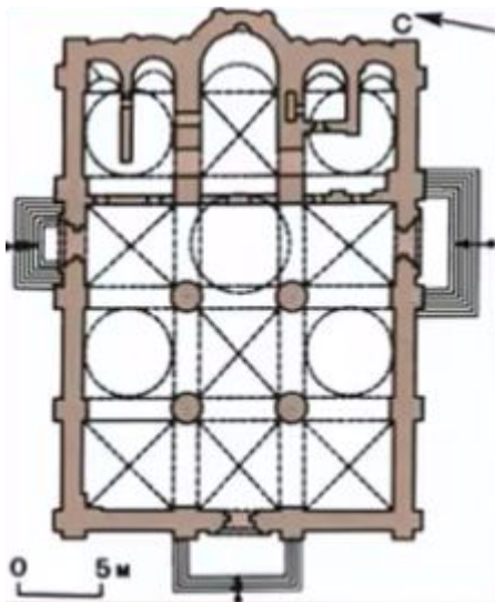
Успенский собор Московского Кремля. План.
