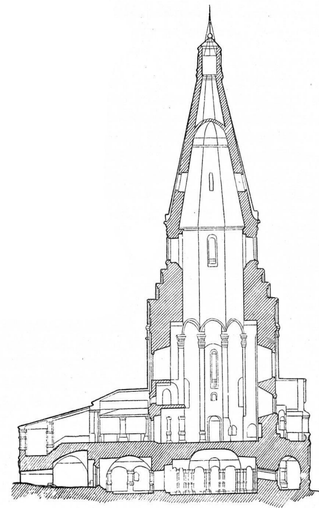
Церковь Вознесения в Коломенском. Продольный разрез
