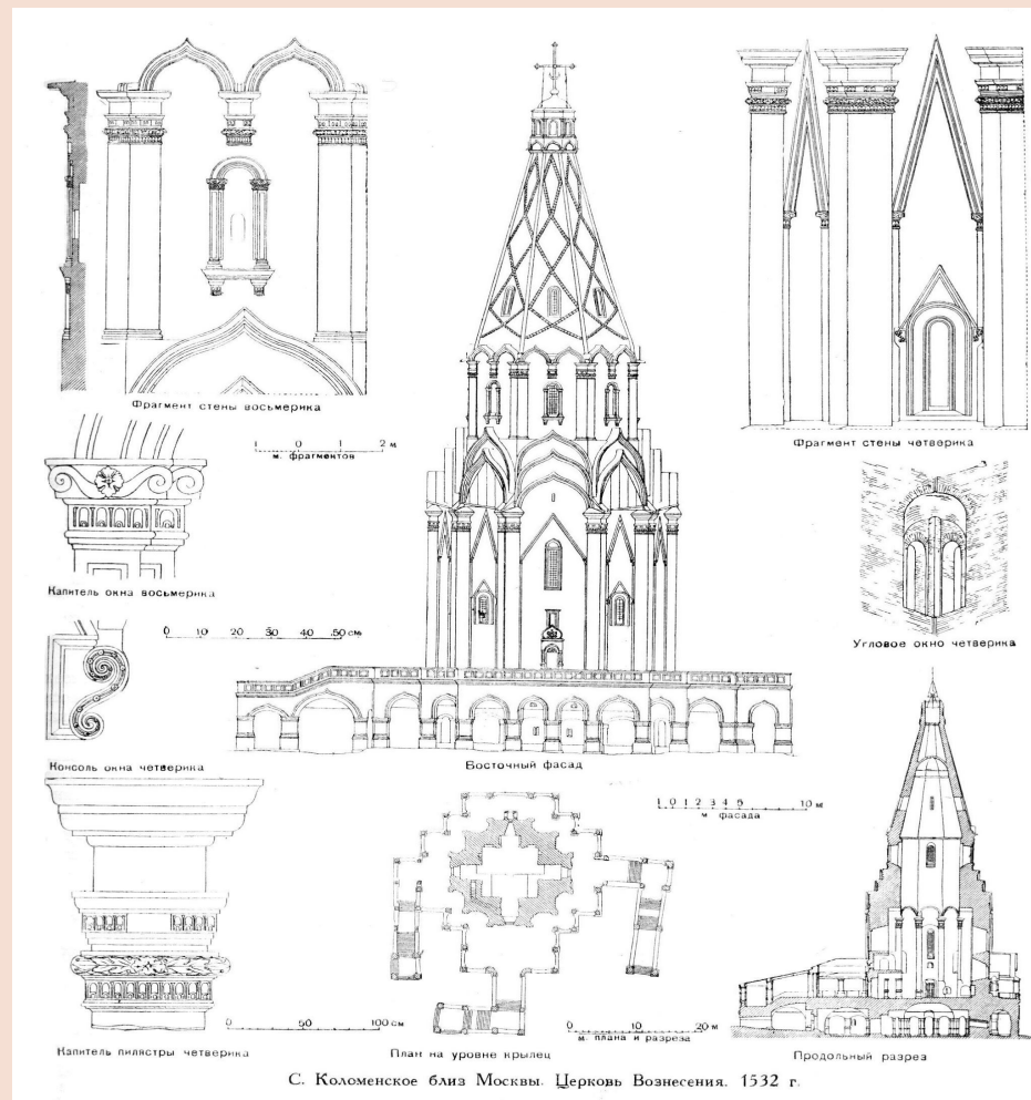
Москва. Церковь Вознесения в Коломенском. 1532 г. Разрез
