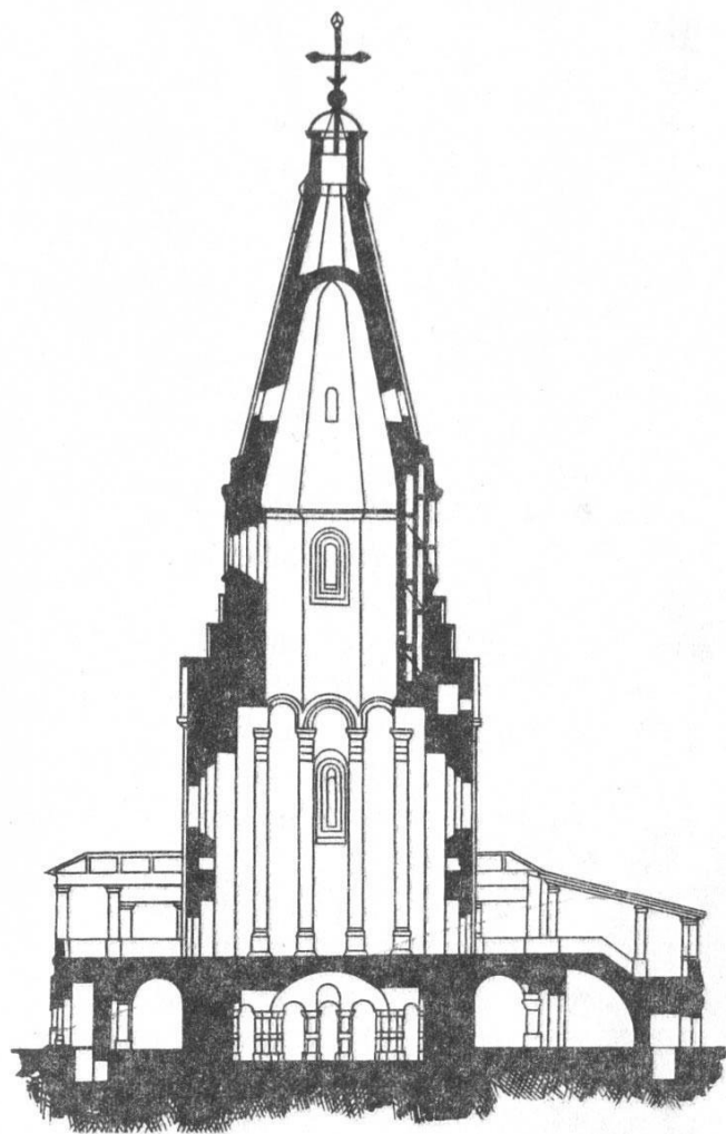
Москва. Церковь Вознесения в Коломенском. 1532 г. Разрез
