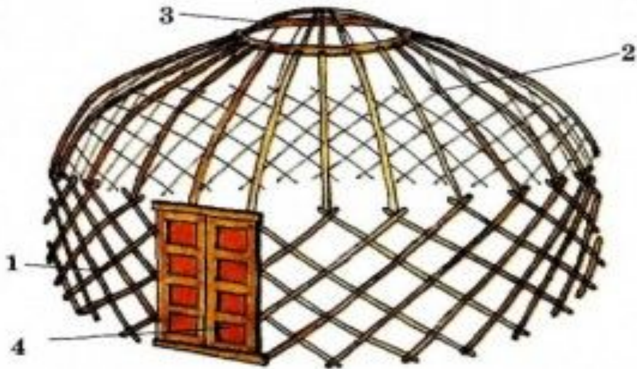
Киіз үйдің сүйегі: 1 – кереге, 2 – уық, 3 – шаңырақ, 4 – сықырлауық
