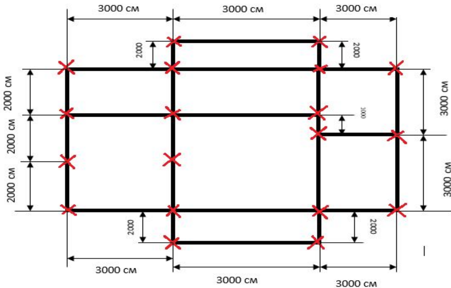
Рис.1 План фундамента
