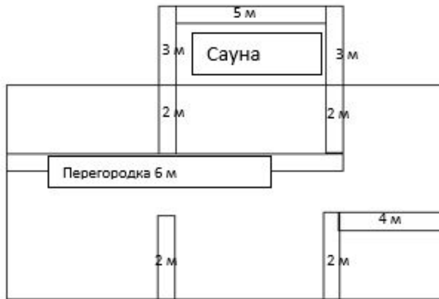
Рис. 3 Расположение перегородок 1 этажа
